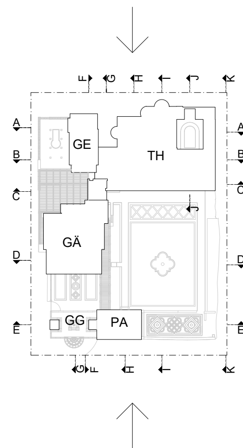
LPH 5 - Ausführungsplanung
